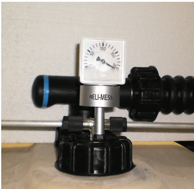
Einbau im Bereich der Flanschen der Entnahmeleitungen Passt Immer
